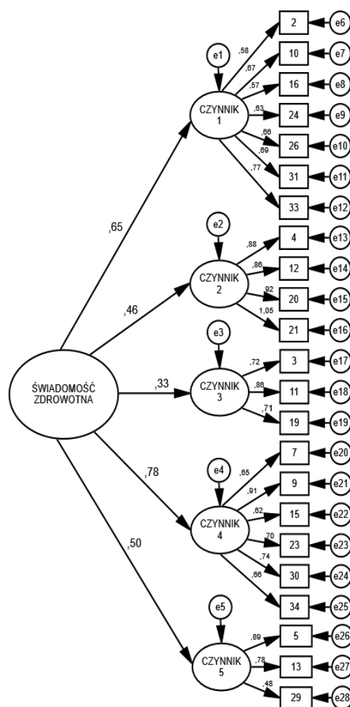
Ryc. 1. Konfirmacyjna analiza czynnikowa ze standardową estymacją
